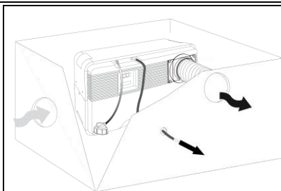
Spillvärmerör och avgasslang via sidoväggen
