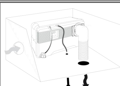
Spillvärmerör och avgasslang via botten
